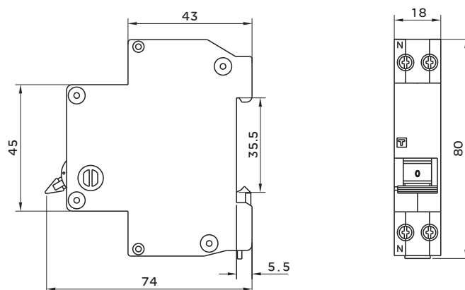
漏电断路器的外形、安装尺寸图
